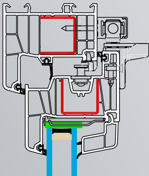
Secțiune verticală fereastră
