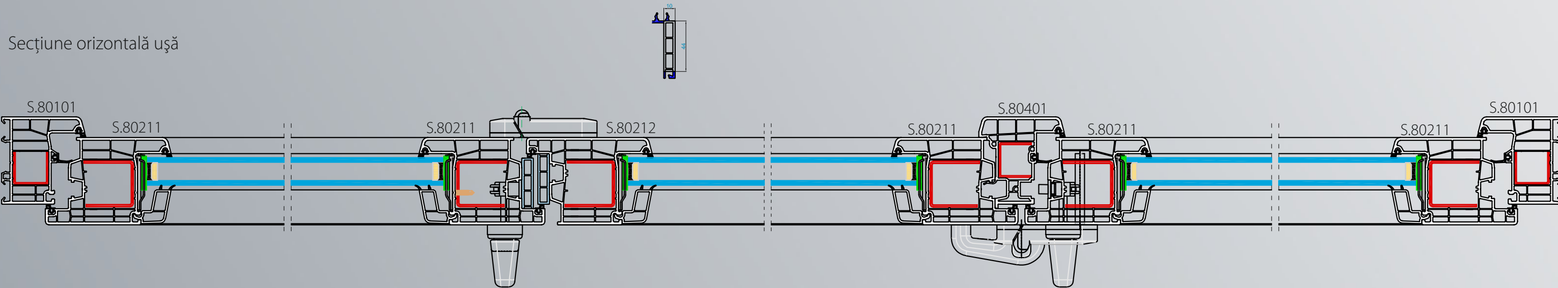
Scheme uși armonice
