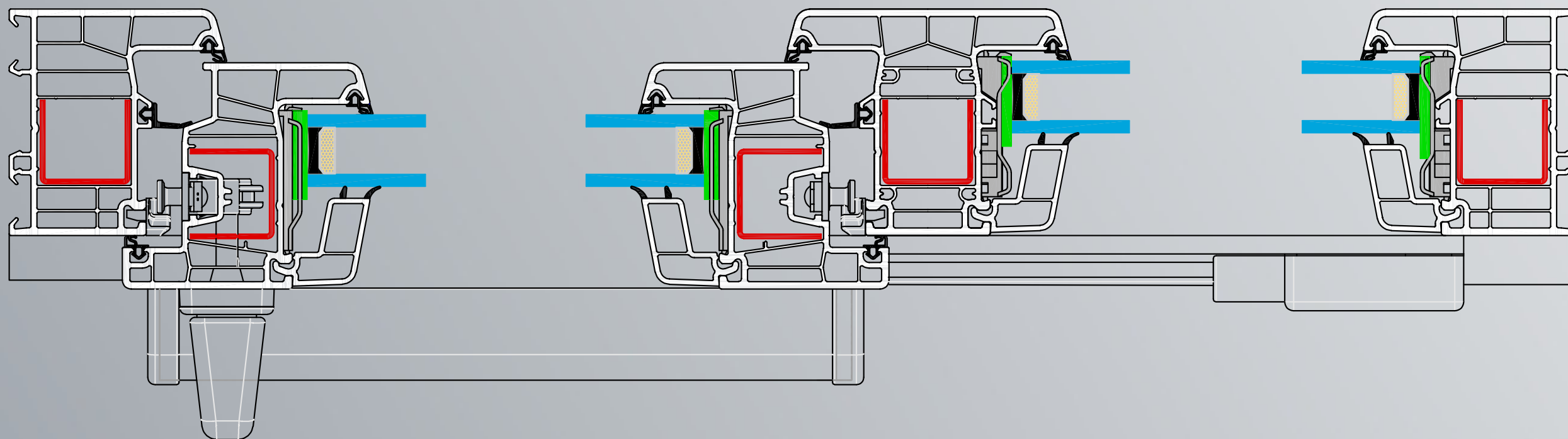
Secțiune orizontală fereastră
