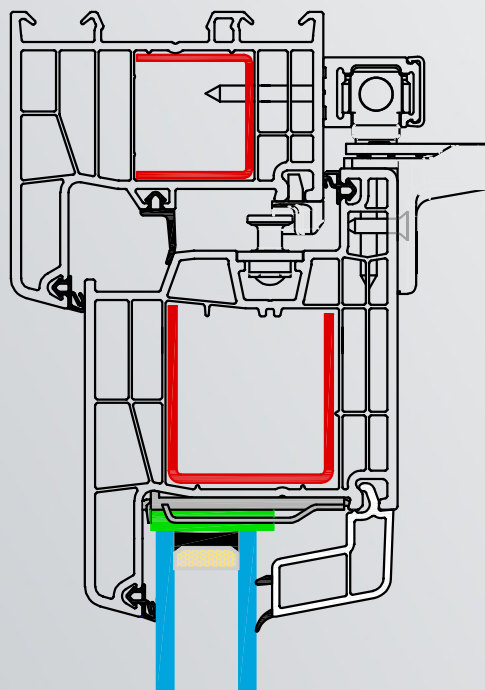
Secțiune verticală ușă
